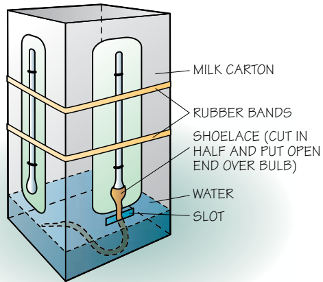
Wet-bulb hygrometer
